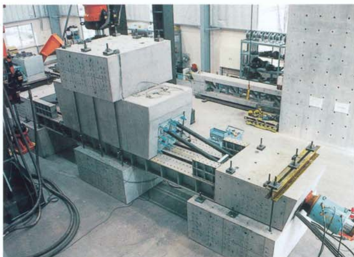
エクストラロード橋サドル部実物大試験
